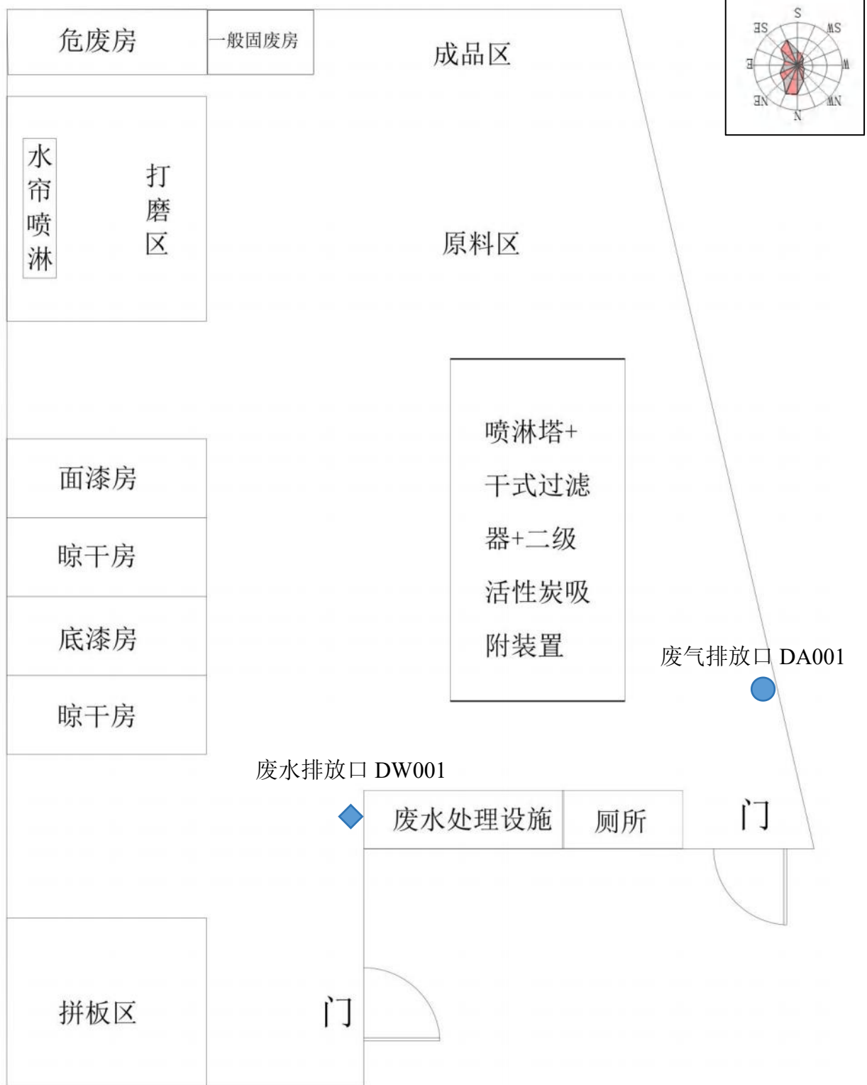
附图 4 总平面布置图
