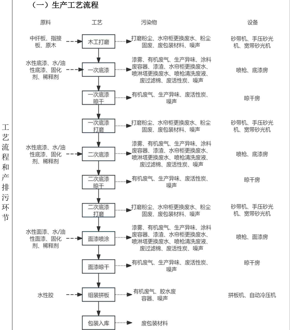
图 5-1 生产工艺流程与产污分析图
